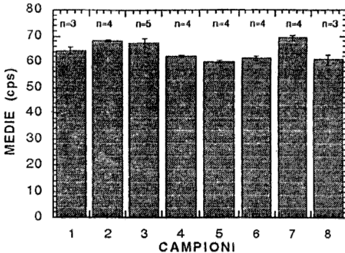
RISPOSTE DIFFRATTOMETRICHE DI 8 SOSPENSIONI DI CRISOSTILO
